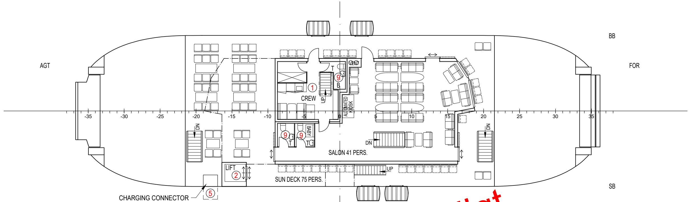
SUN DECK 9000 AB.BL.
